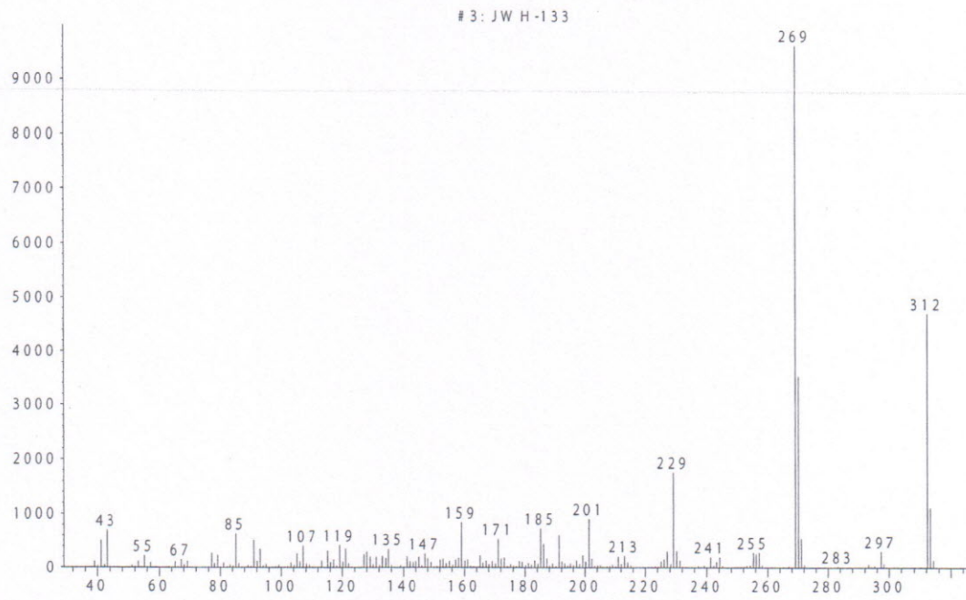
Рис. 3. Масс-спектр "JWH-133"
