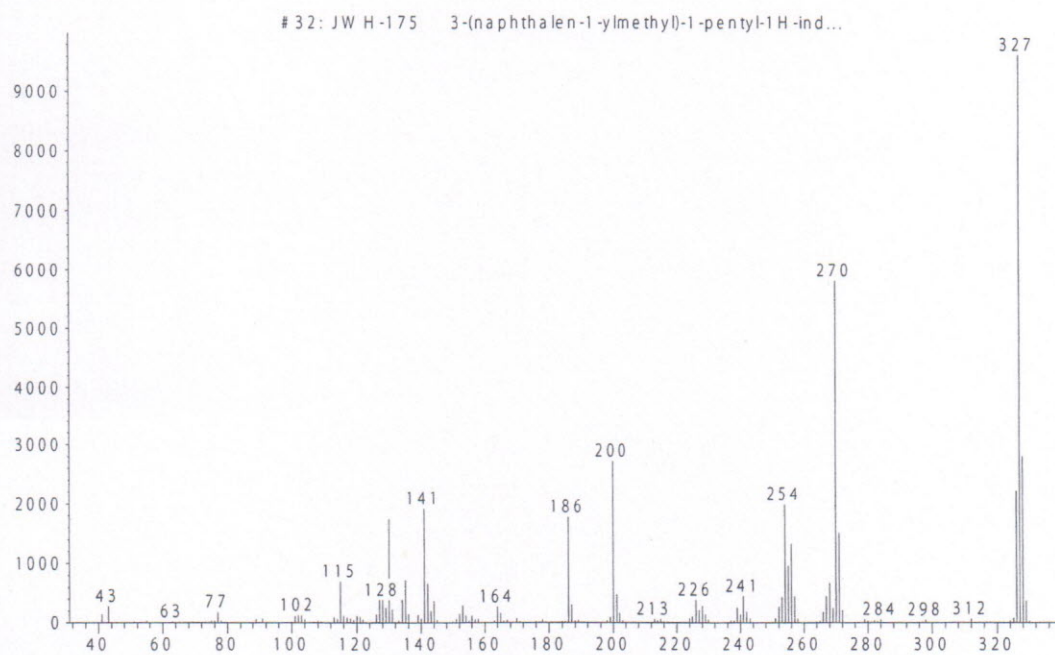
Рис. 8. Масс-спектр "JWH-175"
