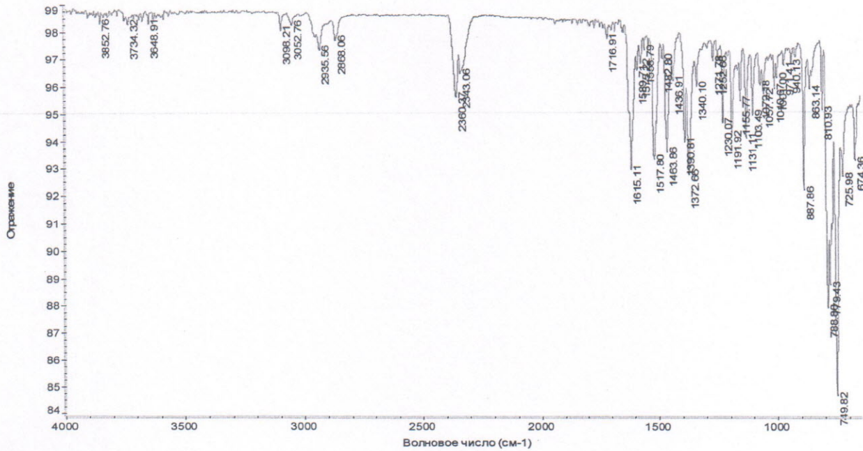
Рис. 25. ИК-спектр JWH-018
