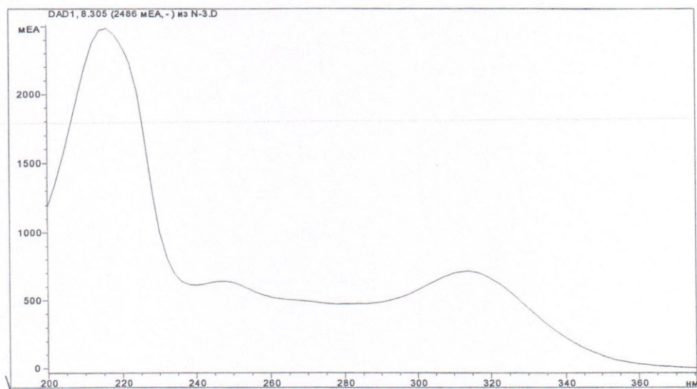
Рис. 21. УФ-спектр вещества «JWH-018» (8.3 мин)
