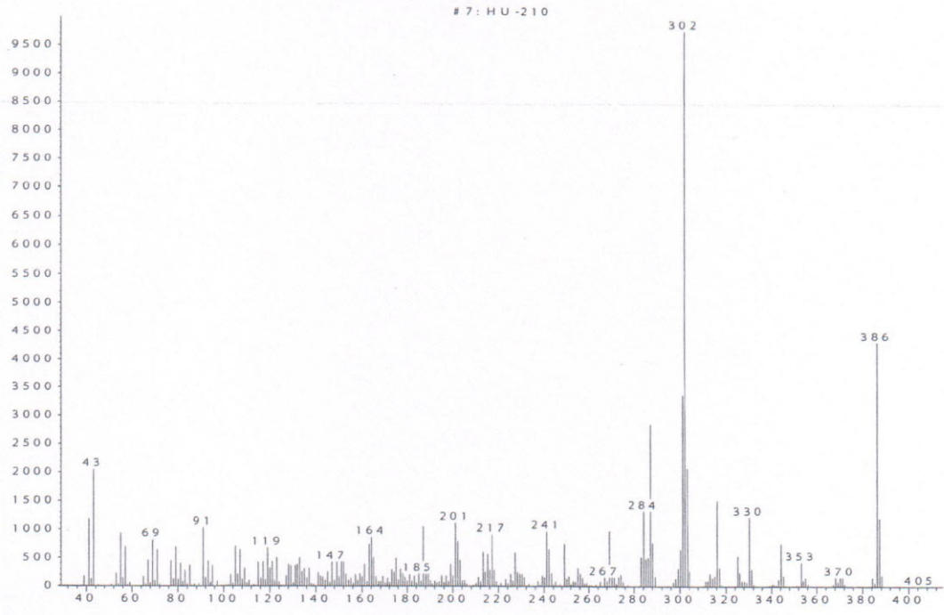
Рис. 13. Масс-спектр "HU-210"
