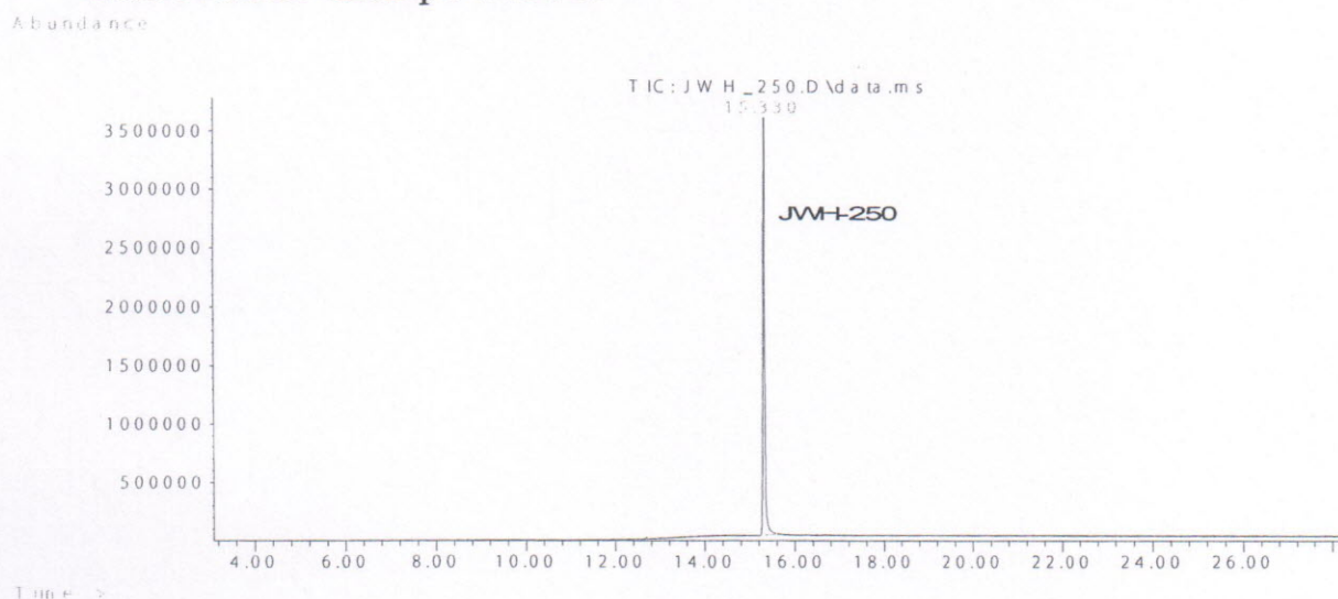
Рис. 10. Хроматограмма курительной смеси «Diamond», содержащей в своём составе JWH-250
