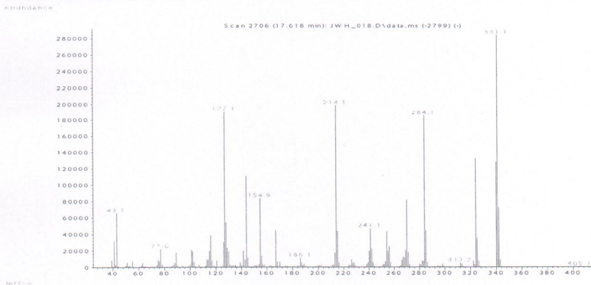
Рис. 2. Масс-спектр пика JWH 018 на спектрограмме исследуемого вещества
