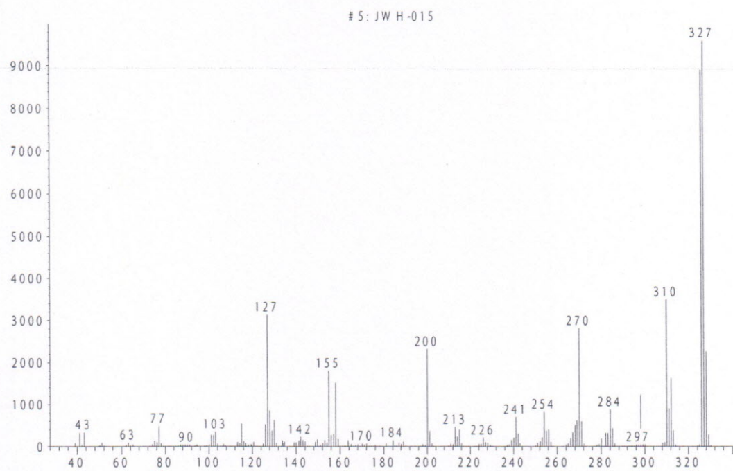
Рис. 5. Масс-спектр "JWH-015"
