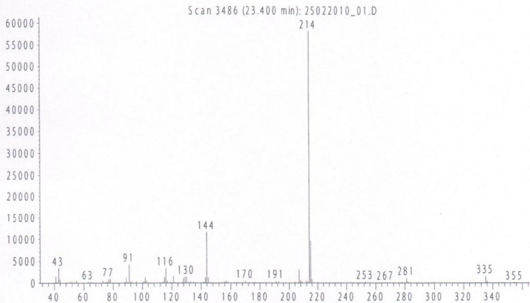
Рис. 10. Масс-спектр "JWH-250"
