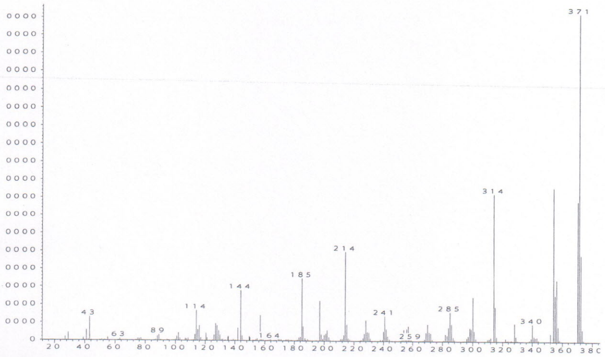
Рис. 11. Масс-спектр "JWH-081"
