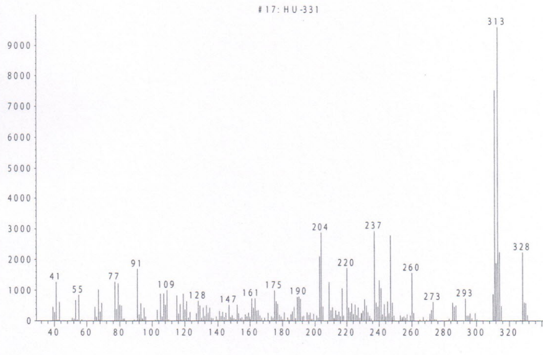
Рис. 13. Масс-спектр "HU-331"
