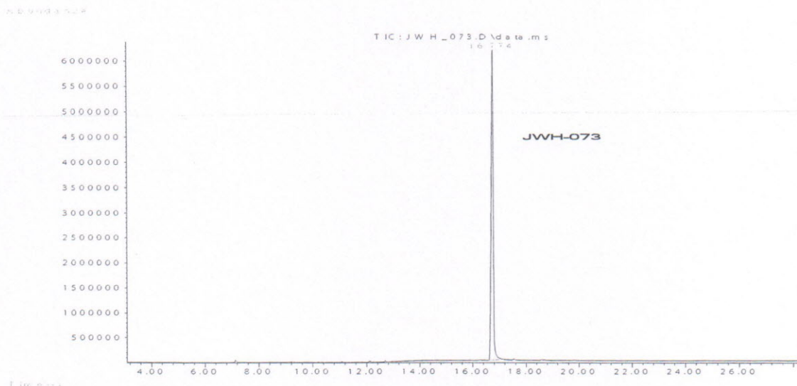
Рис. 6. Хроматограмма курительной смеси «Jah Rush POWER», содержащей в своём составе JWH-073
