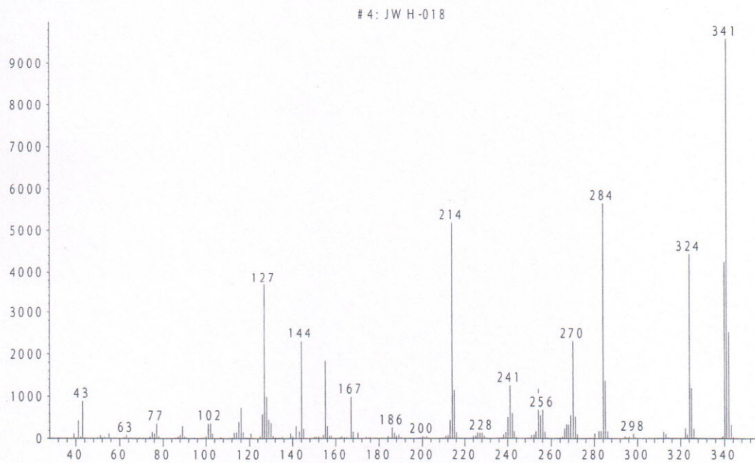
Рис. 4. Масс-спектр "JWH-018"
