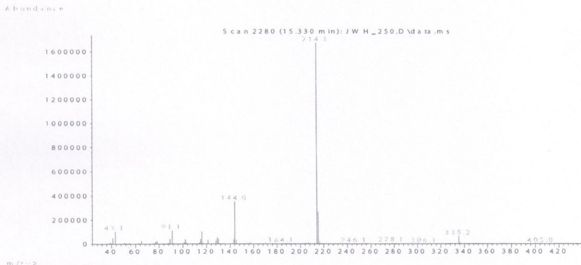
Рис. 11. Масс-спектр JWH-250
