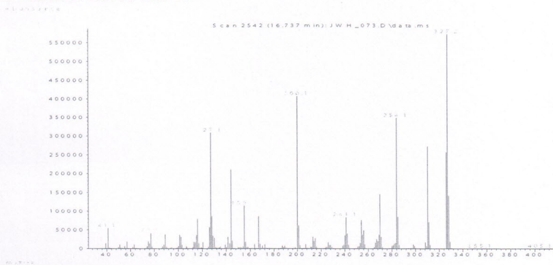
Рис. 7. Масс-спектр пика JWH-073 на спектрограмме исследуемого вещества
