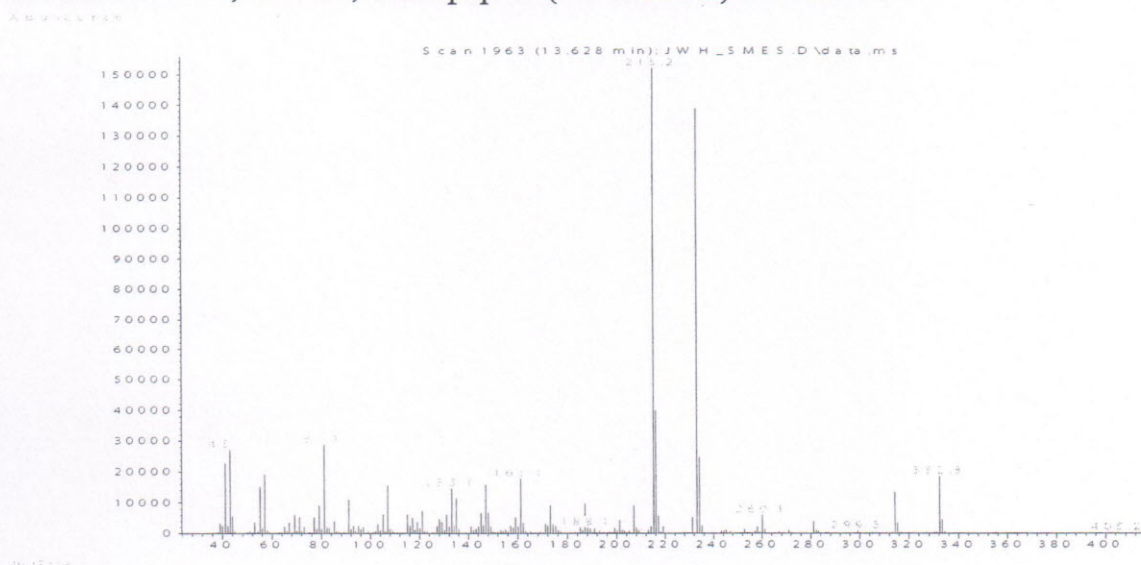
Рис. 4 Масс-спектр Z-изомера CP 47,497-C8 (цис-диастереомер)
