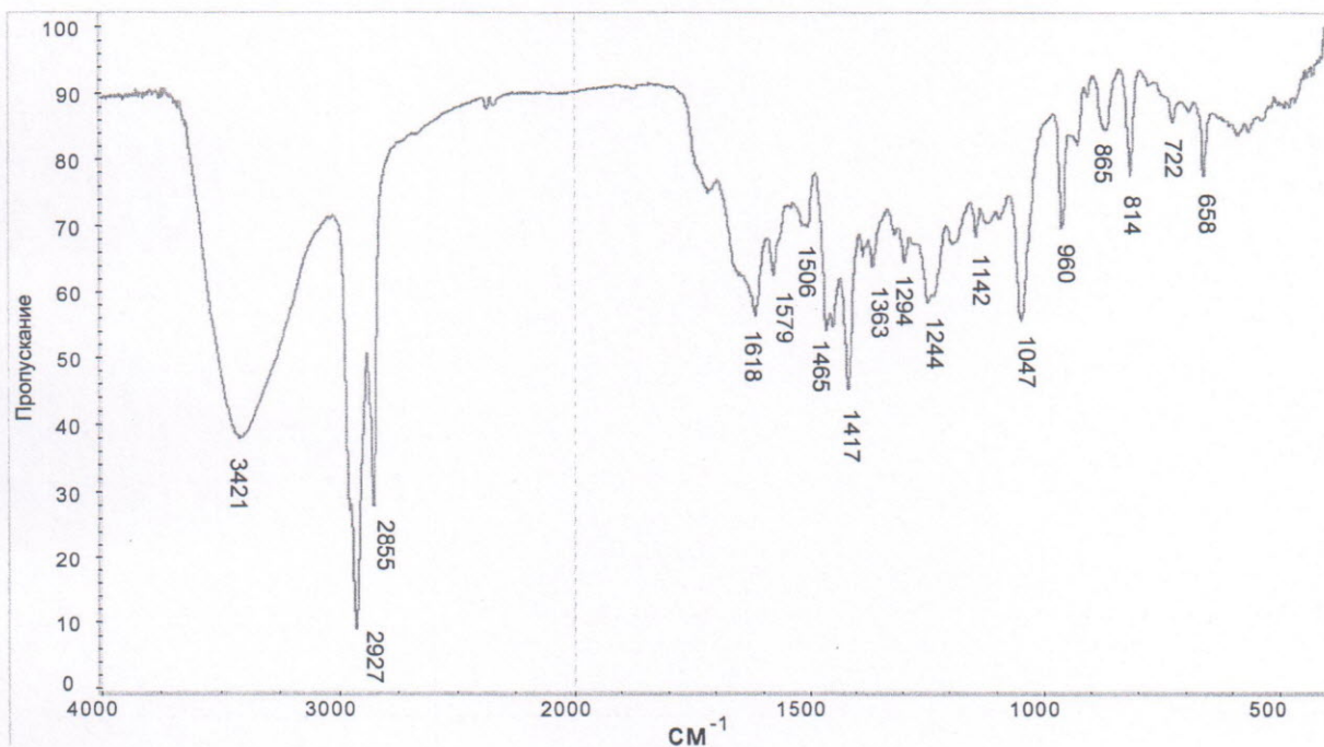
Рис. 26. ИК-спектр JWH-073
