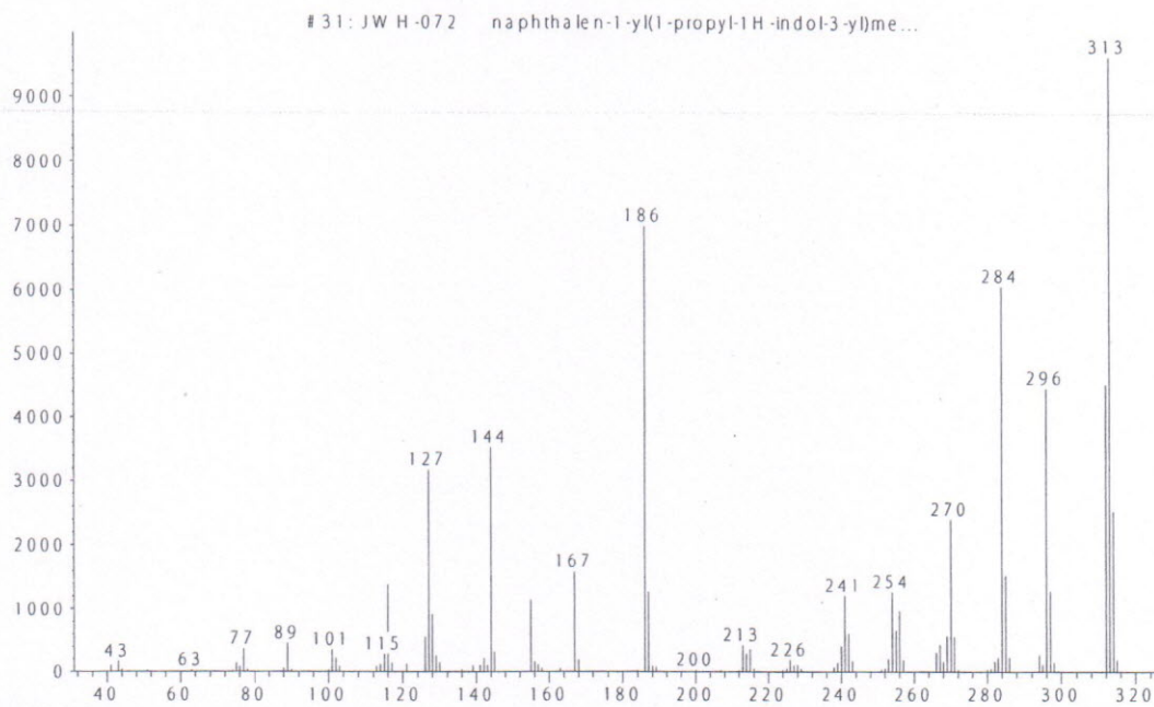
Рис. 7. Масс-спектр "JWH-072"
