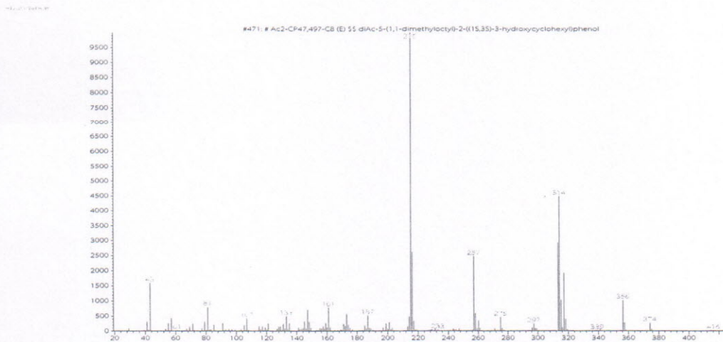
Рис. 13. Масс-спектр диацетильного производного E -изомера «СР 47,497-С8»
