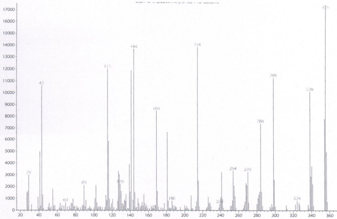
Рис. 12. Масс-спектр "JWH-122"
