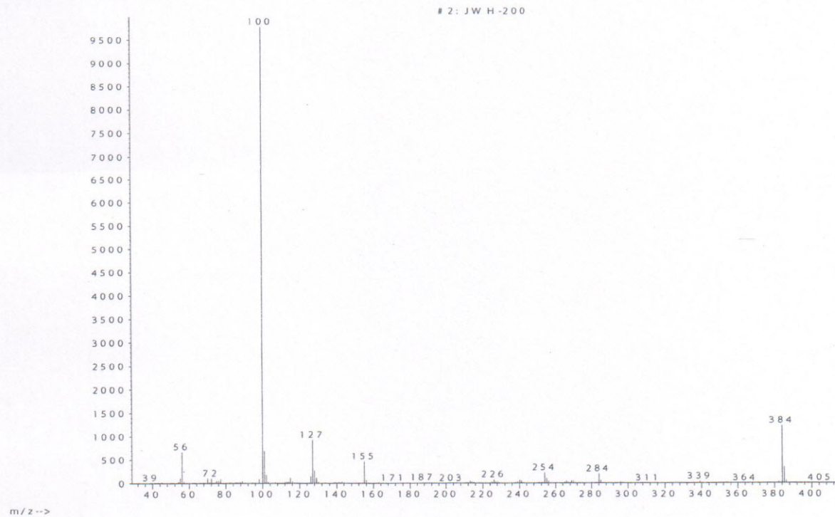
Рис. 2. Масс-спектр "JWH-200"
