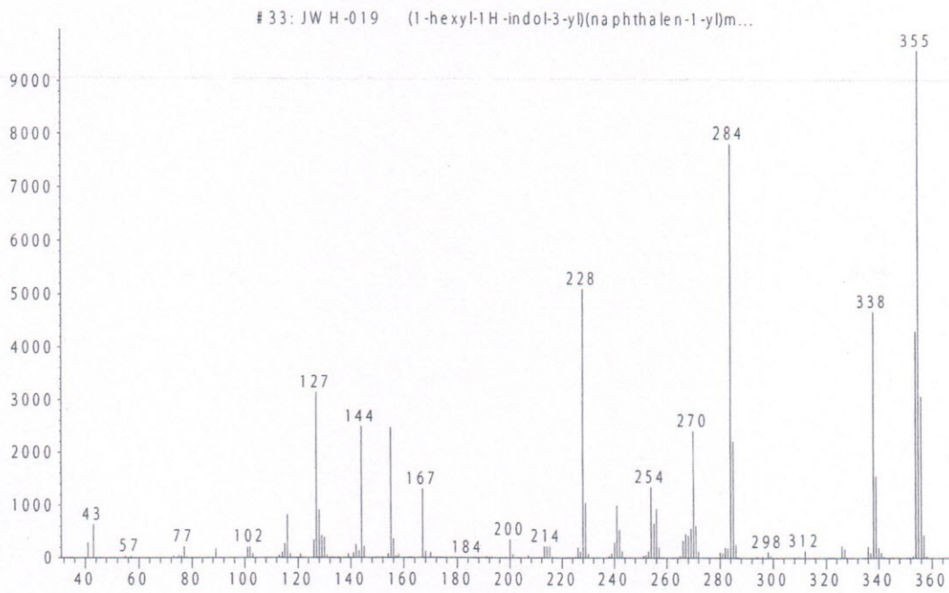
Рис. 9. Масс-спектр "JWH-019"
