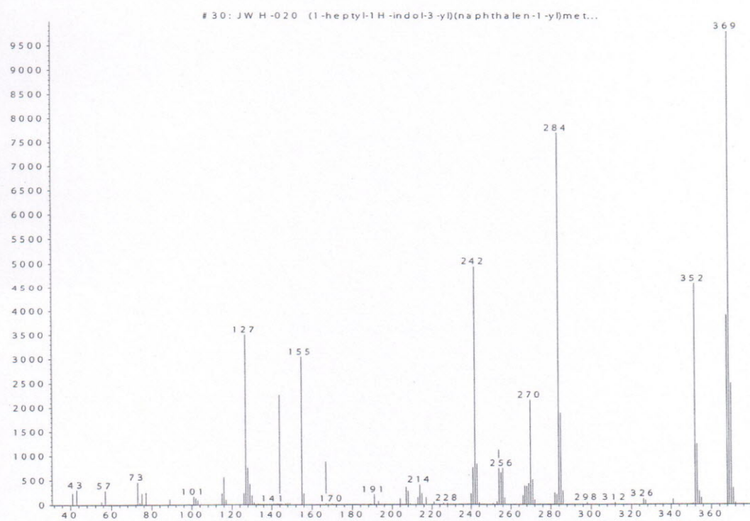
Рис. 6. Масс-спектр "JWH-020"
