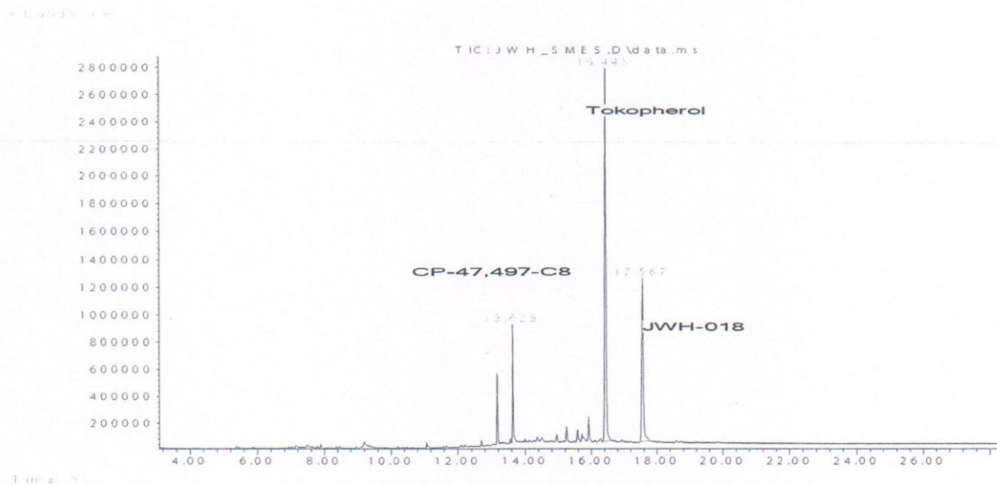
Рис. 3. Хроматограмма курительной смеси «Spice», содержащей в своём составе CP 47,497-C8, токоферол (витамин E) и JWH-018
