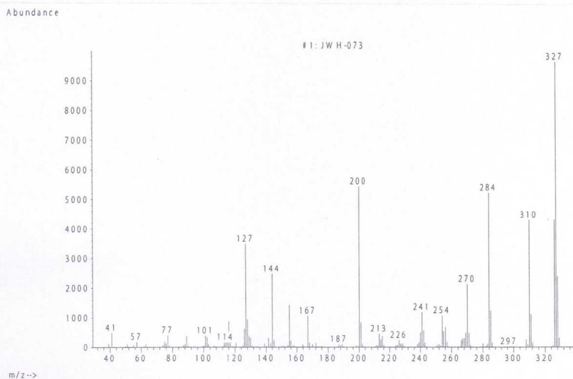
Рис. 1. Масс-спектр "JWH-073"
