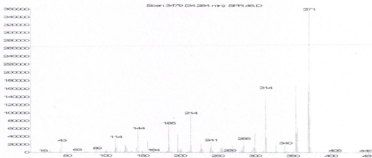
Рис. 9. Масс-спектр JWH-081
